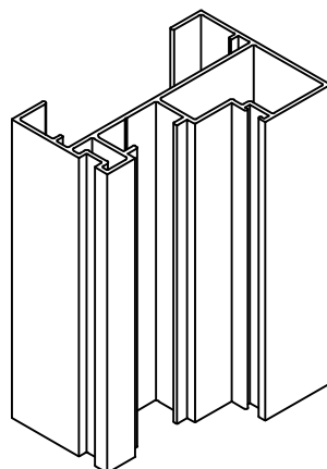
Huisserie ref: EVO400
